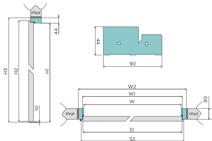
OŚCIEŻNICA STAŁA DREWNIANA SUROWA
