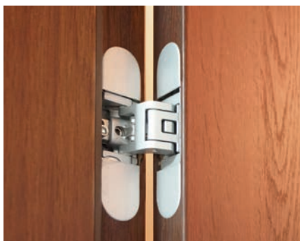
ZAWIAS WPUSZCZANY Z REGULACJĄ W TRZECH PŁASZCZYZNACH
